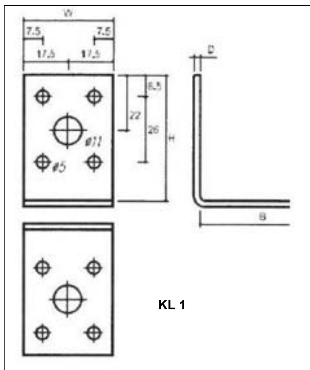
Rysunek 17 Typ KL
