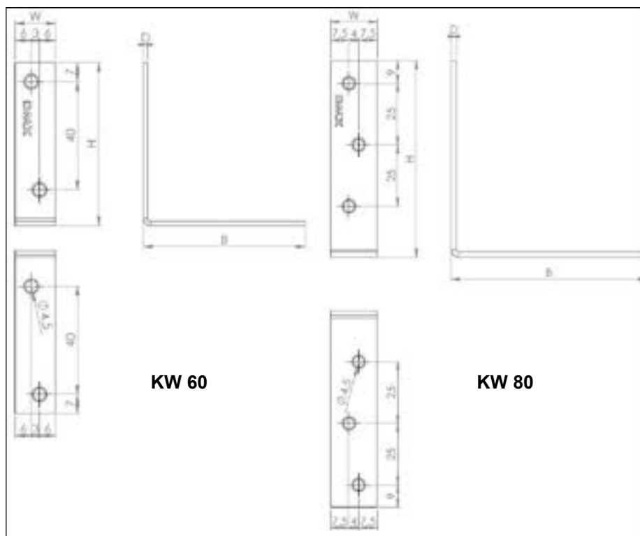
Rysunek 57 Typ KW
