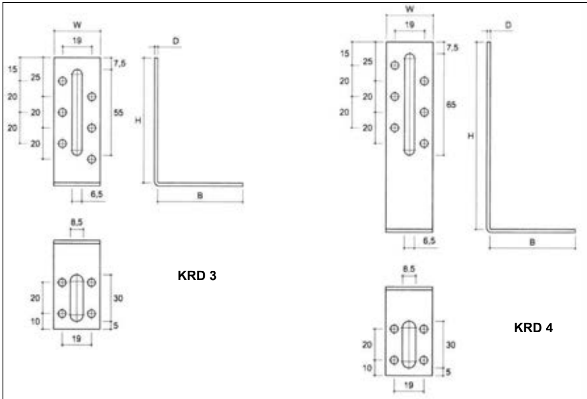
Rysunek 8 Typ KRD
