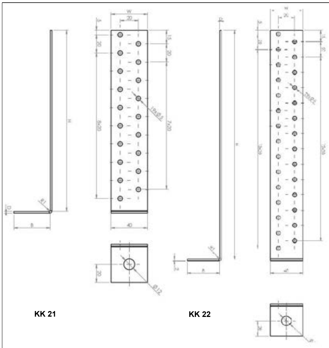
Rysunek 15 Typ KK
